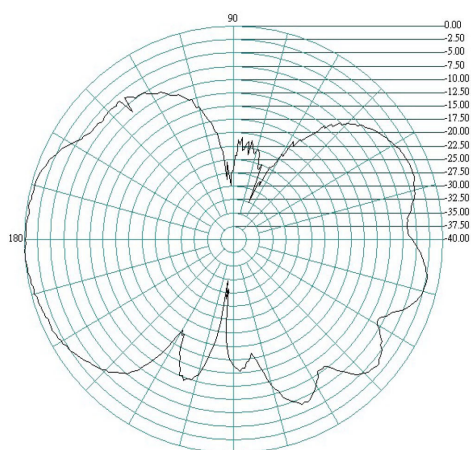
E-PLANE
