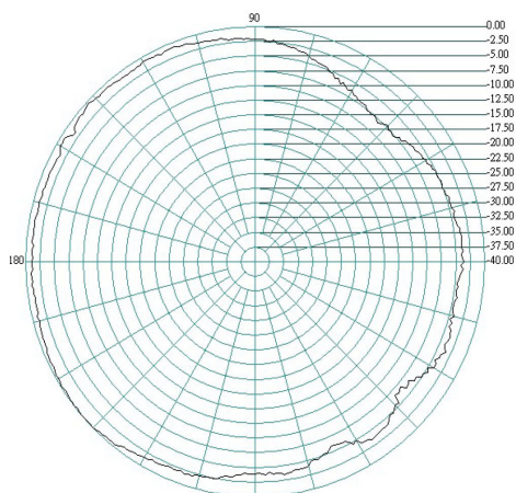
H-PLANE
