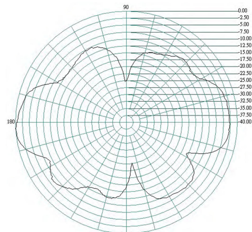
E-PLANE
