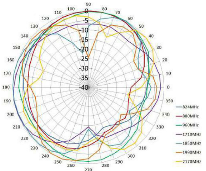
E-PLANE
