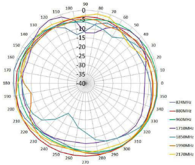
H-PLANE
